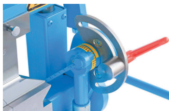
Biegewinkelbegrenzungsanschlag (Serienausstattung)
