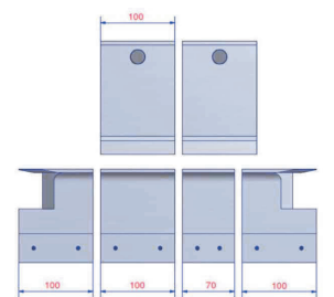
Fensterbankeinsatz Variabel
