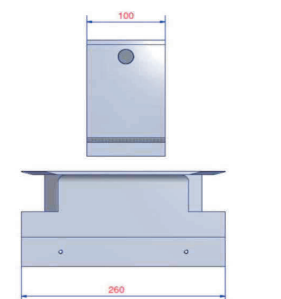
Fensterbankeinsatz Standard
